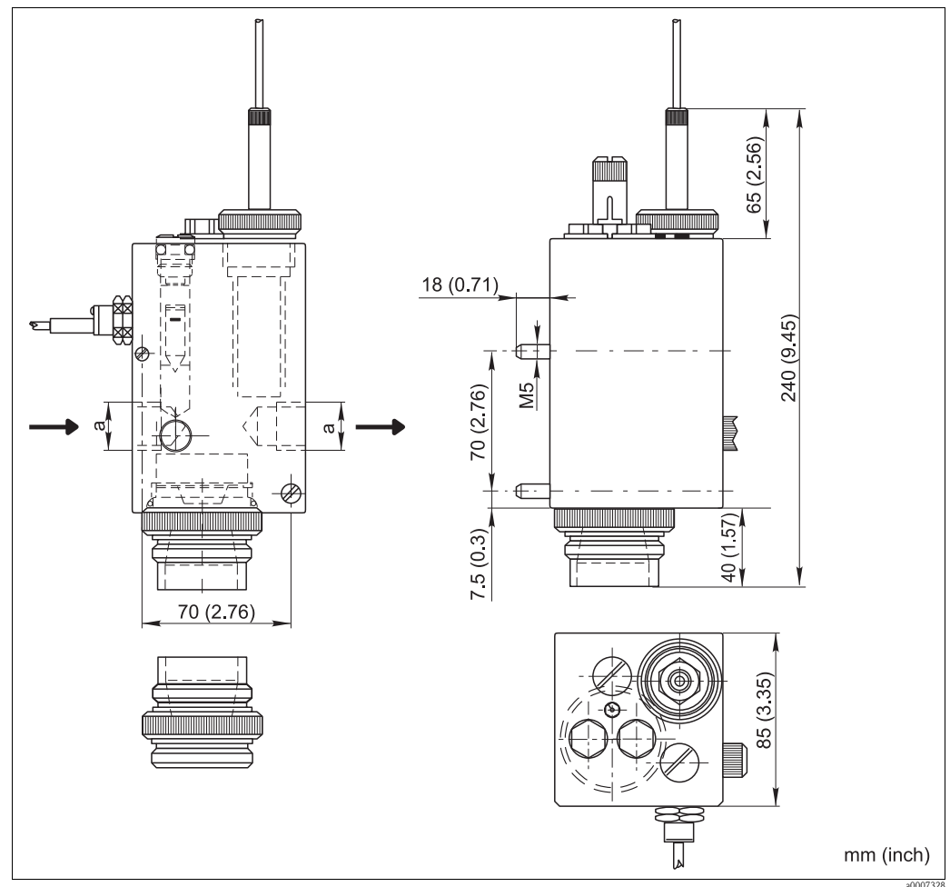
Fig. 2: Dimensions
