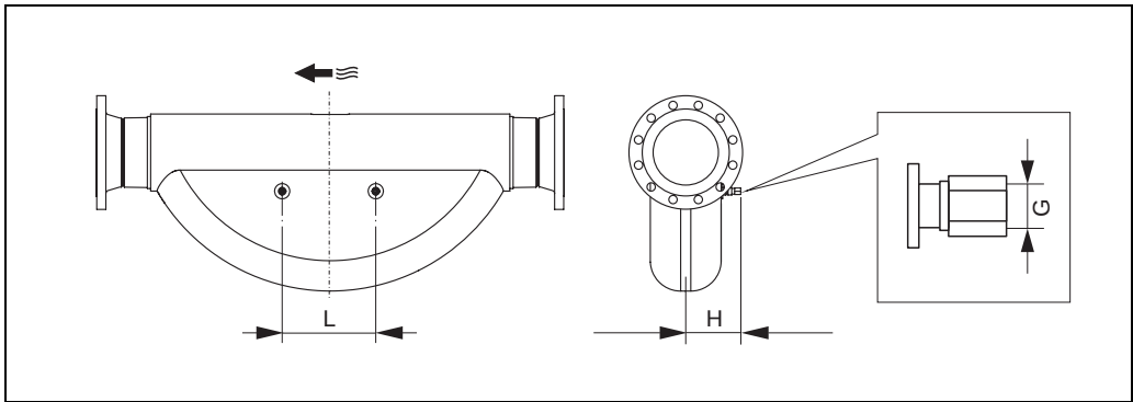
DN 250 (10")
