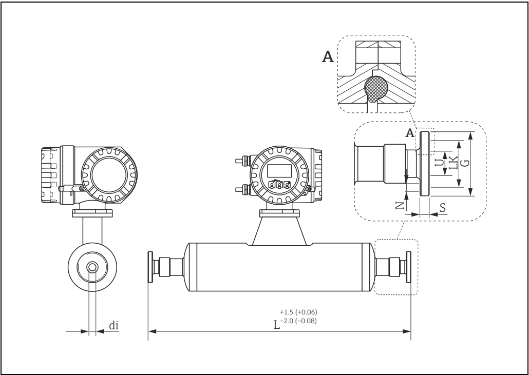
DIN 11864-2A flange, DIN 11866 line A, flange with notch
